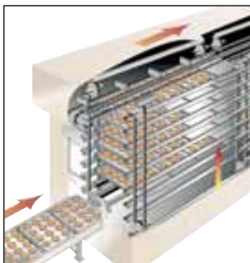
Formenlogistik Flexibles Lager für Doppellinie
